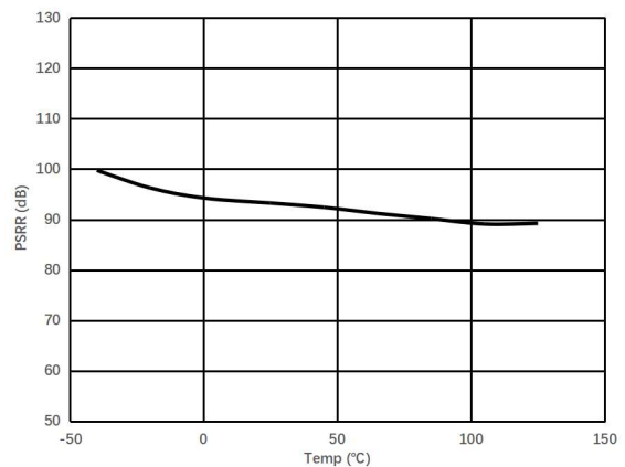
图 1.7.12. 直流 PSRR 与温度的关系 @ V_S = 1.6\text{V} 到 5.5\text{V}
