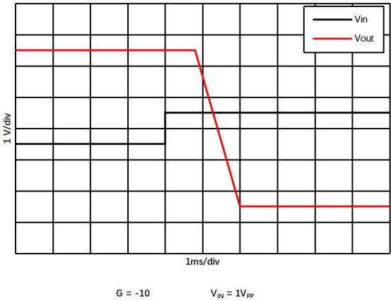
图 1.9.7. 正过载恢复
