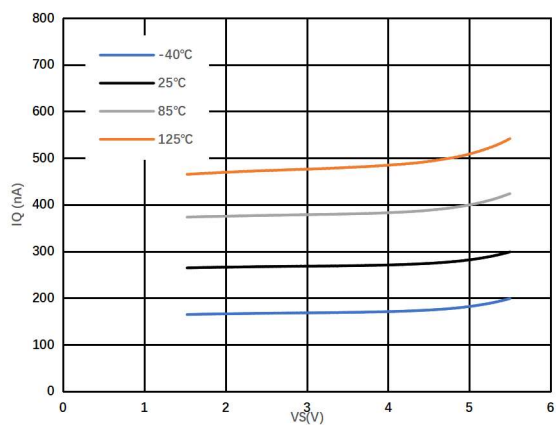
图 1.7.4. 静态电流 vs 供电电压 @ V_{CM} = 0\text{V} (SID103D/Q)
