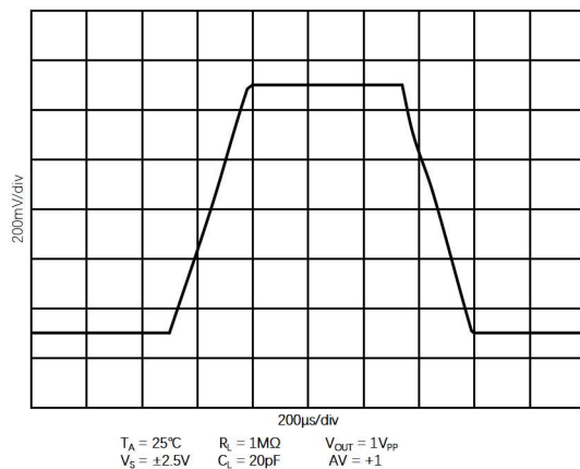
图 1.9.3. 大信号阶跃响应 @ V_S = 5\text{V}
