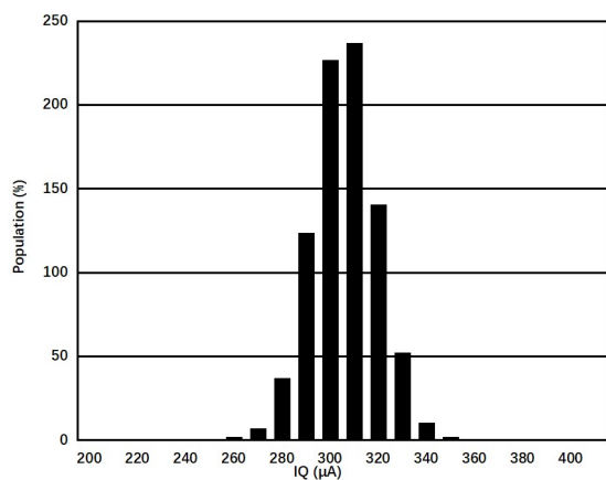
图 1.7.3. 静态电流分布图 (SID103D/Q)
