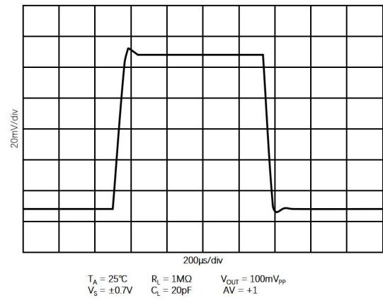
图 1.9.2. 小信号阶跃响应 @ V_S = 1.4\text{V}
