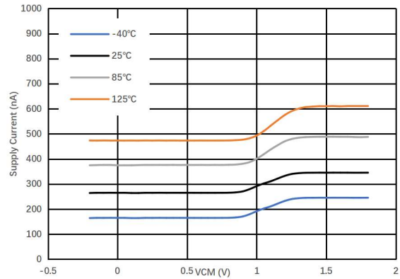
图 1.7.8. 静态电流 vs 共模电压 @ V_S = 1.6\text{V} (SID103D/Q)
