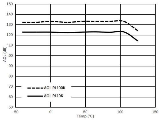
图 1.7.13. 开环增益与温度的关系 @ V_S = 5.0\text{V}
