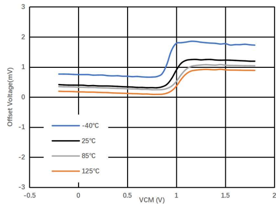
图 1.7.10. 输入失调电压 vs 共模电压 @ V_S = 1.6\text{V}
