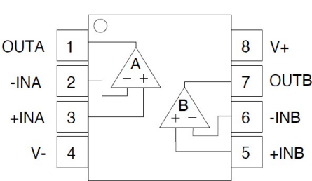
SOP8/MSOP8
