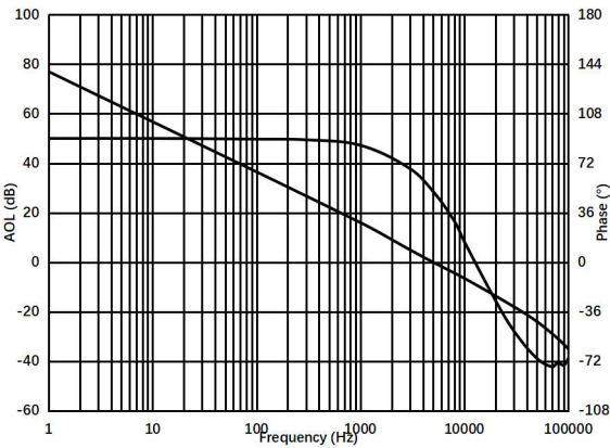
图 1.8.1. 开环增益与相位
