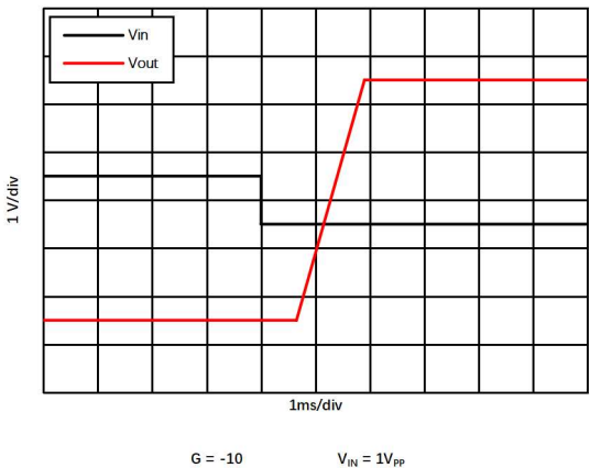
图 1.9.8. 负过载恢复
