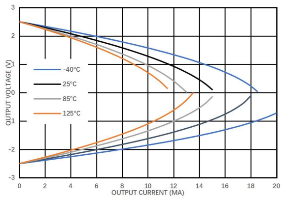
图 1.7.15. 输出电压 vs 输出电流 @ V_S = 5\text{V}
