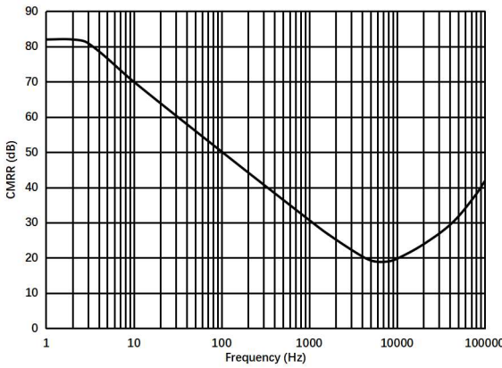
图 1.8.3. CMRR vs 频率
