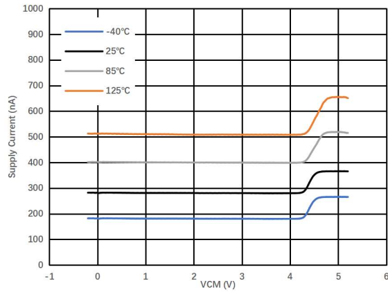
图 1.7.7. 静态电流 vs 共模电压 @ V_S = 5\text{V} (SID103D/Q)
