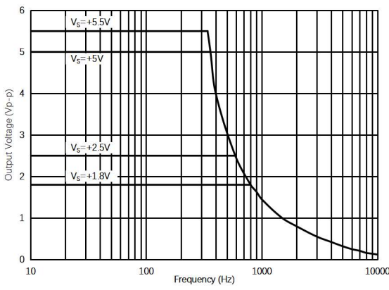
图 1.8.4. 最大输出电压 vs 频率
