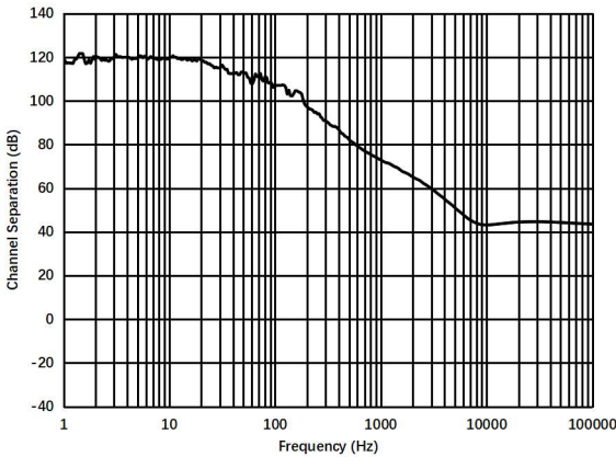
图 1.10.1. 通道隔离度 (SID103D/Q)
