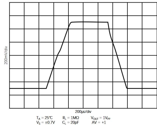
图 1.9.4. 大信号阶跃响应 @ V_S = 1.4\text{V}
