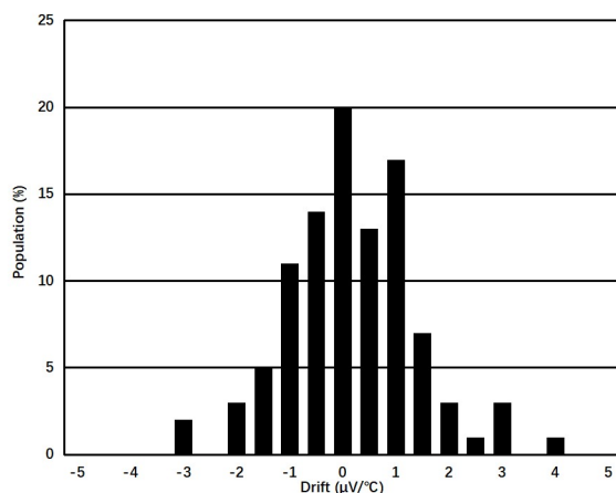
图 1.7.2. 温漂分布图
