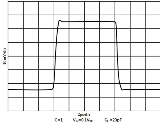
图 1.9.1. 小信号阶跃响应 @ V_S = 5\text{V}
