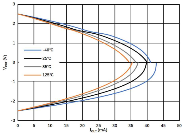
图 1.7.15. 输出电压 vs 输出电流 @ V_S = 5\text{V}
