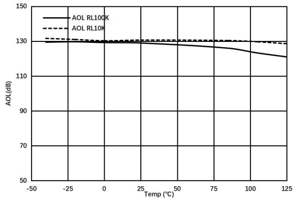
图 1.7.13. 开环增益与温度的关系 @ V_S = 5.0\text{V}
