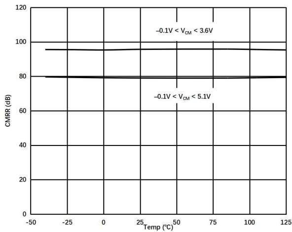
图 1.7.11. 直流 CMRR 与温度的关系 @ V_S = 5\text{V}
