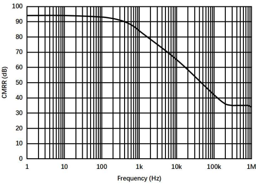
图 1.8.2. PSRR vs 频率
