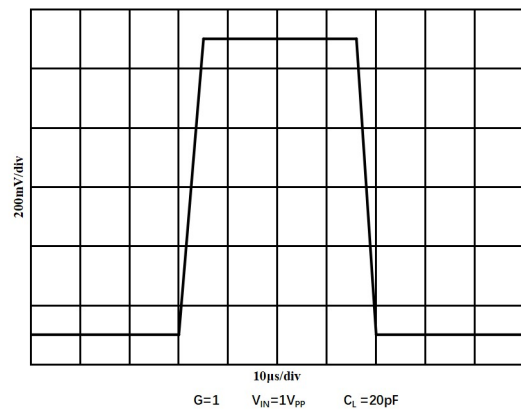
图 1.9.4. 大信号阶跃响应 @ V_S = 1.8\text{V}
