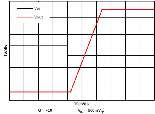
图 1.9.8. 负过载恢复
