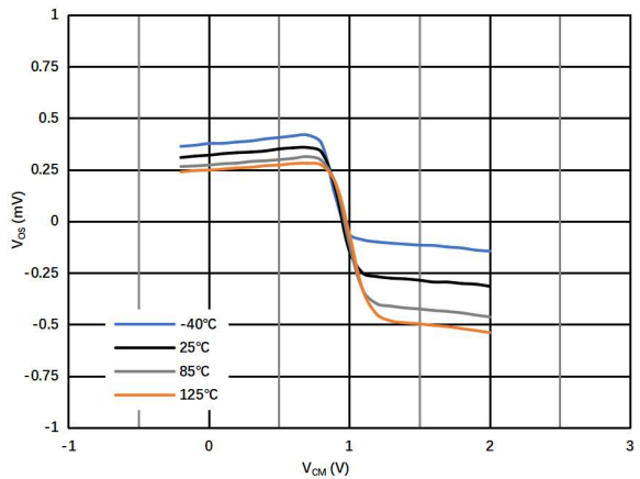
图 1.7.10. 输入失调电压 vs 共模电压 @ V_S = 1.8\text{V}
