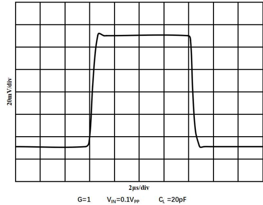
图 1.9.2. 小信号阶跃响应 @ V_S = 1.8\text{V}
