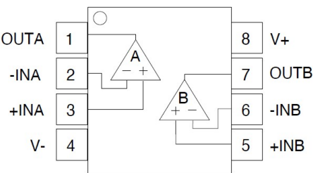
SOP8/MSOP8
