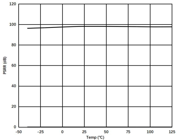
图 1.7.12. 直流 PSRR 与温度的关系 @ V_S = 1.8\text{V} 到 5.5\text{V}
