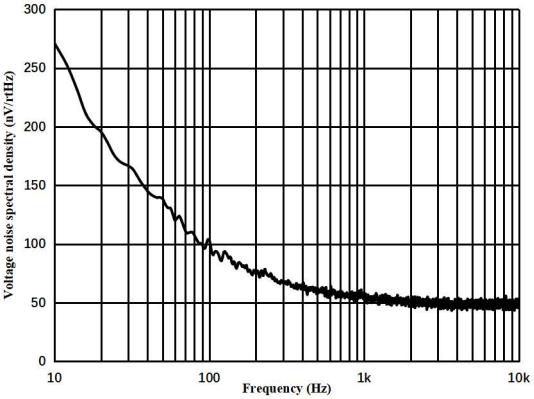
图 1.8.6. 输入电压噪声频谱密度
