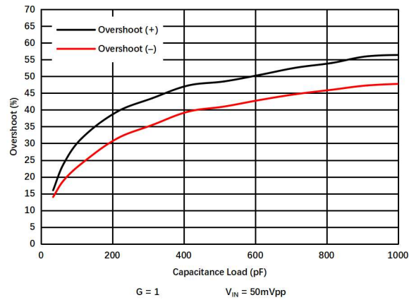
图 1.9.9. 小信号过冲与容性负载
