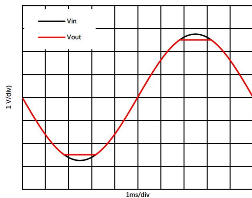
图 1.9.5. 无相位翻转
