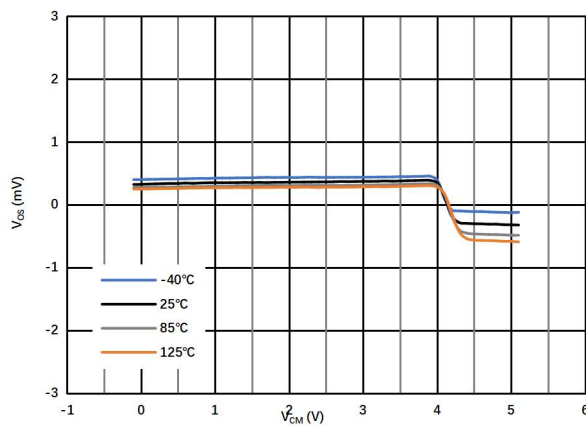
图 1.7.9. 输入失调电压 vs 共模电压 @ V_S = 5\text{V}
