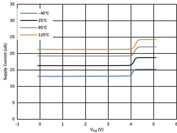
图 1.7.7. 静态电流 vs 共模电压 @ V_S = 5\text{V}
