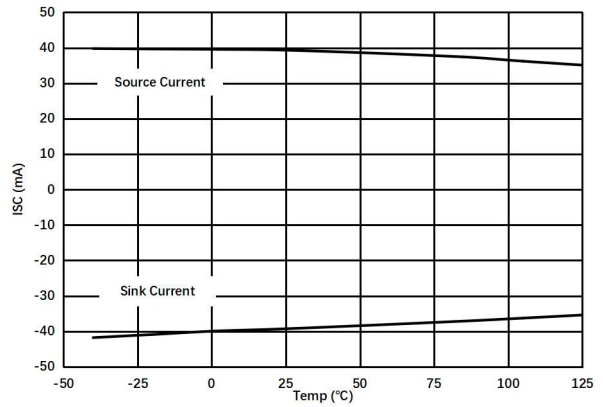
图 1.7.14. 输出短路电流与温度的关系 @ V_S = 5\text{V}
