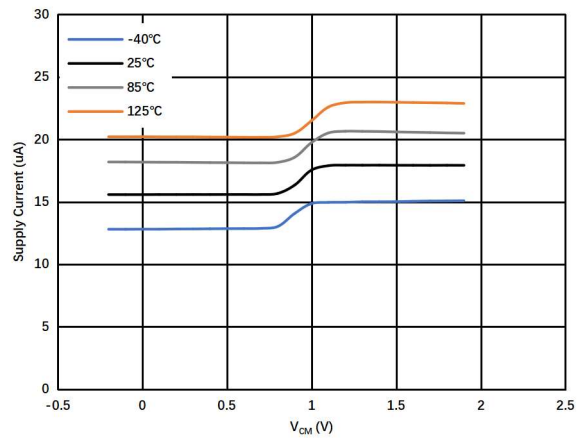
图 1.7.8. 静态电流 vs 共模电压 @ V_S = 1.8\text{V}
