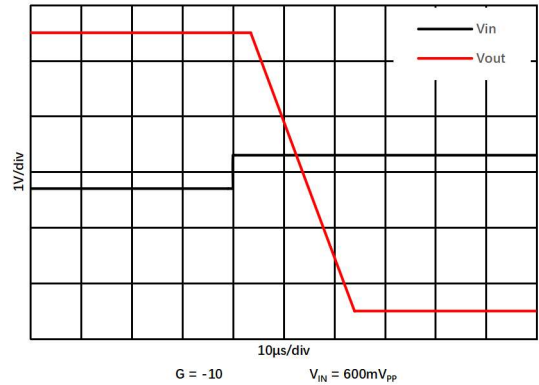
图 1.9.7. 正过载恢复
