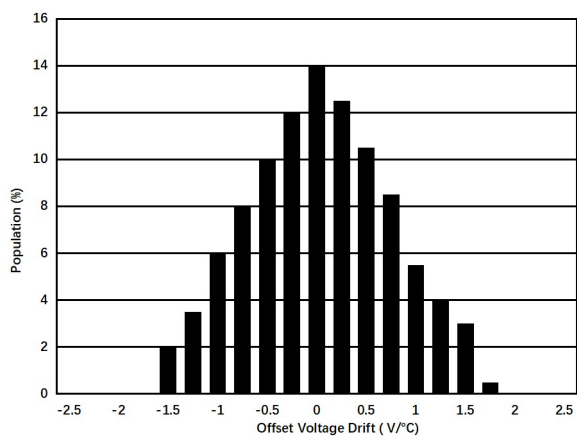
图 1.7.2. 温漂分布图
