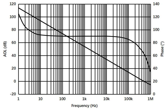
图 1.8.1. 开环增益与相位
