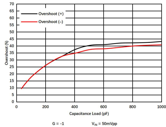
图 1.9.10. 小信号过冲与容性负载
