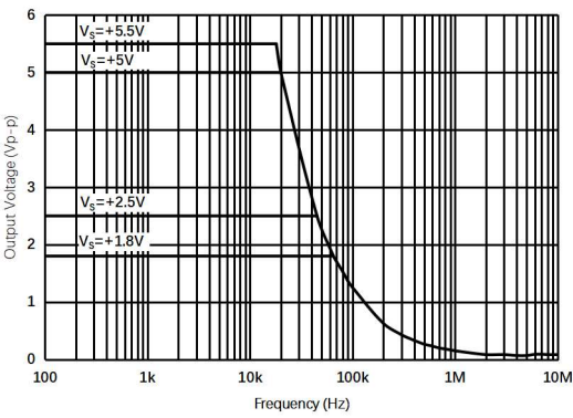
图 1.8.4. 最大输出电压 vs 频率
